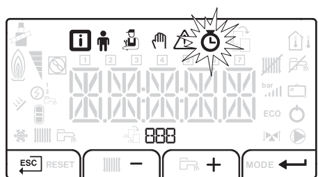
Afb.32 Submenu-parameters weergeven TELLER
