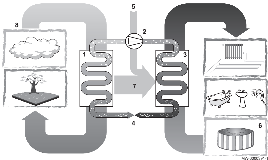
Afb.3 Algemeen werkingsprincipe
