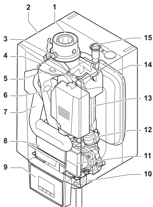
Afb.4 Alezio G hybrid 24/28 MI - 34/39 MI
