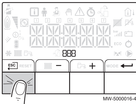
Afb.29 Terug naar het hoofdscherm
