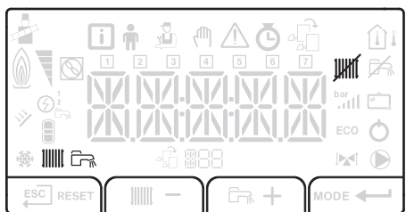
Afb.10 Werkingsmodi
