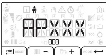
Afb.39 Gebruikersmenu weergeven
