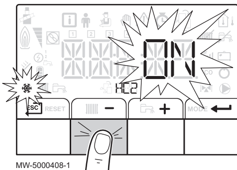
Afb.37 Koelingsmodus bevestigen
