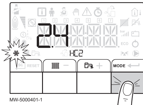
Afb.37 Koelingsmodus bevestigen
