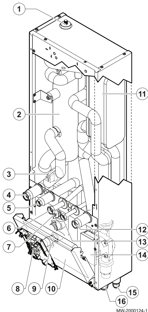
Afb.5 Voornaamste componenten van de hydraulische module
