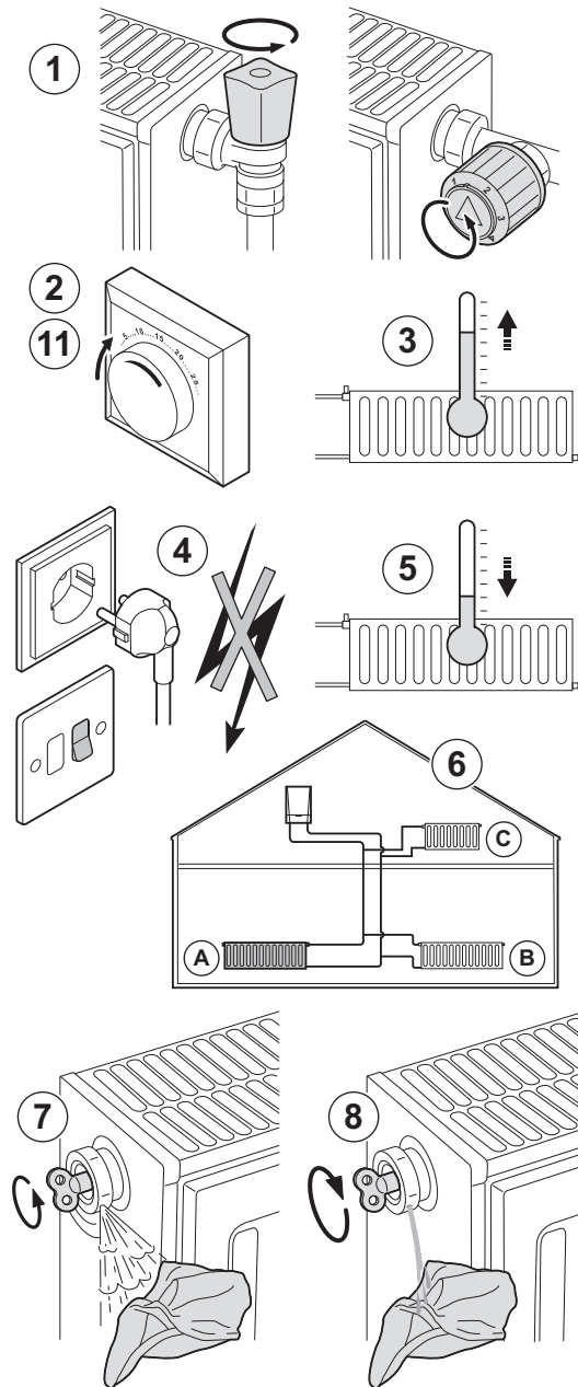
Afb.56 Ontluchten van de installatie
